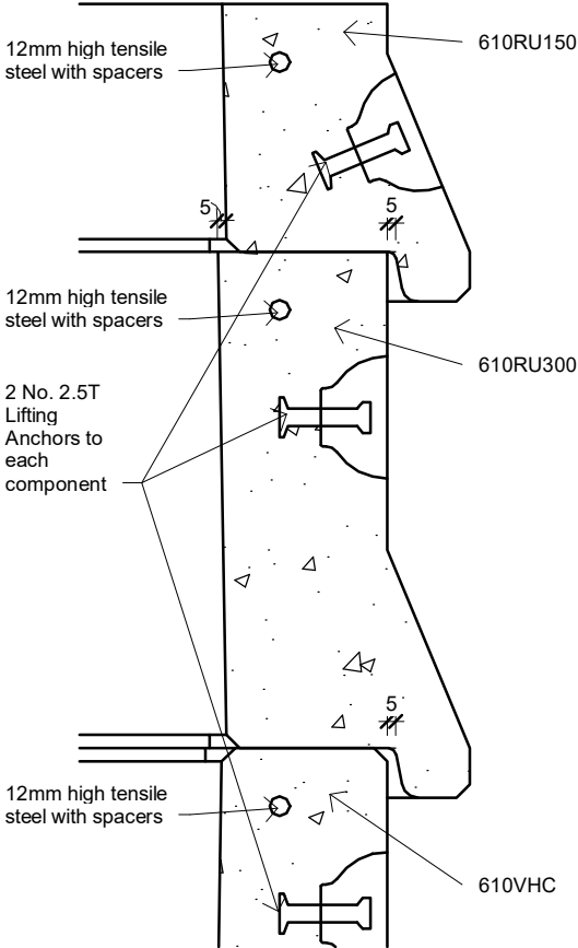
3 Detail 1 1 : 5
