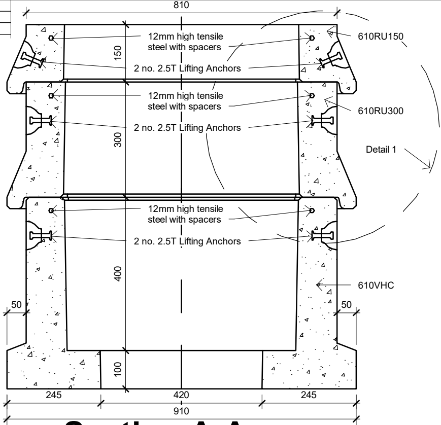
2 Section A-A 1 : 10
