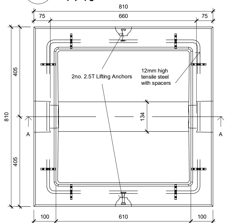
1 Plan 1 : 10
