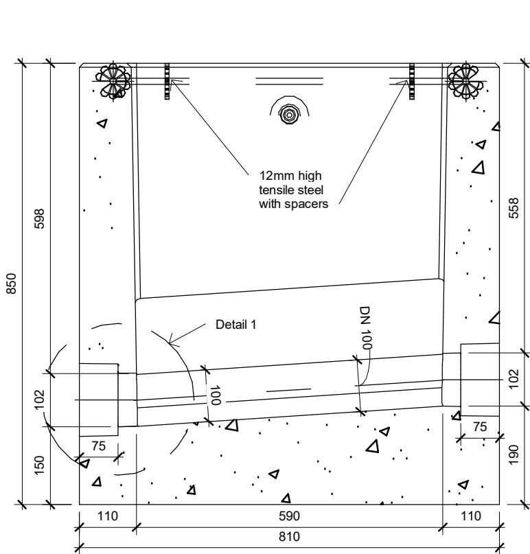
2 Section A-A 1 : 10
