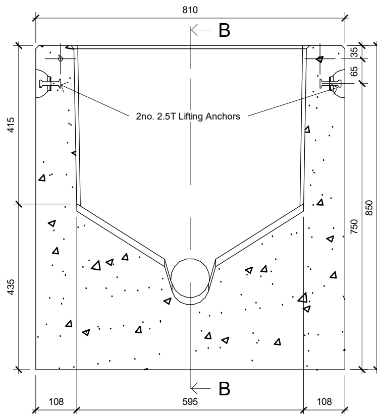
3 Section B-B 1 : 10
