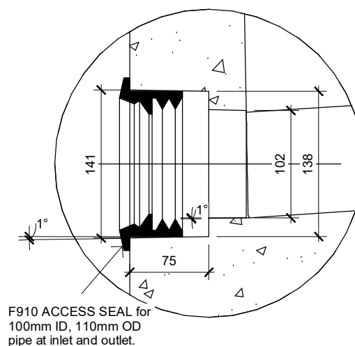
4 Detail 1 1 : 5
