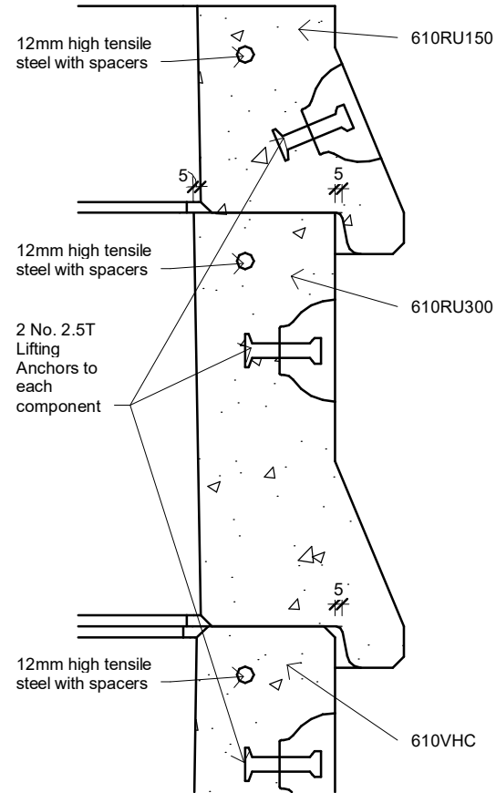
3 Detail 1 1 : 5
