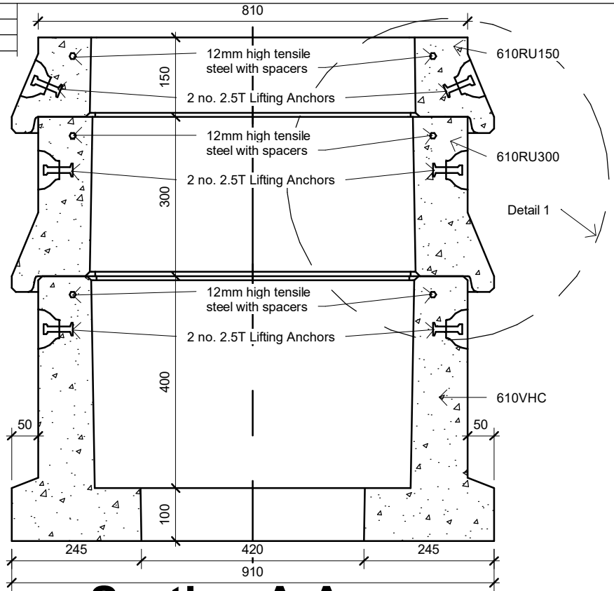
2 Section A-A 1 : 10
