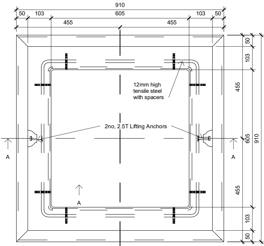
1 Plan 1 : 10
