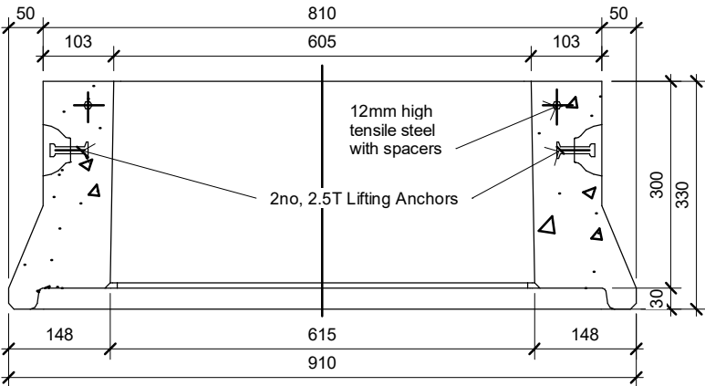
2 Section A-A 1 : 10
