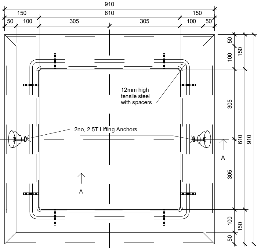
1 Plan 1 : 10
