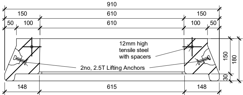
2 Section A-A 1 : 10
