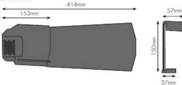
Dimensions
